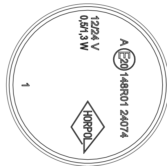
SZCZEGÓŁ C
